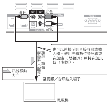
BDP-LX55 的後面板
